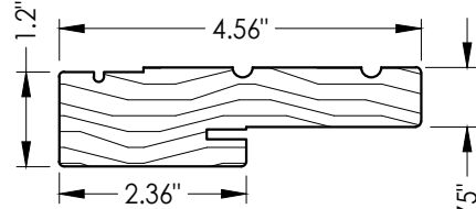
1A WOOD JAMB FrameSaver (Endura)
