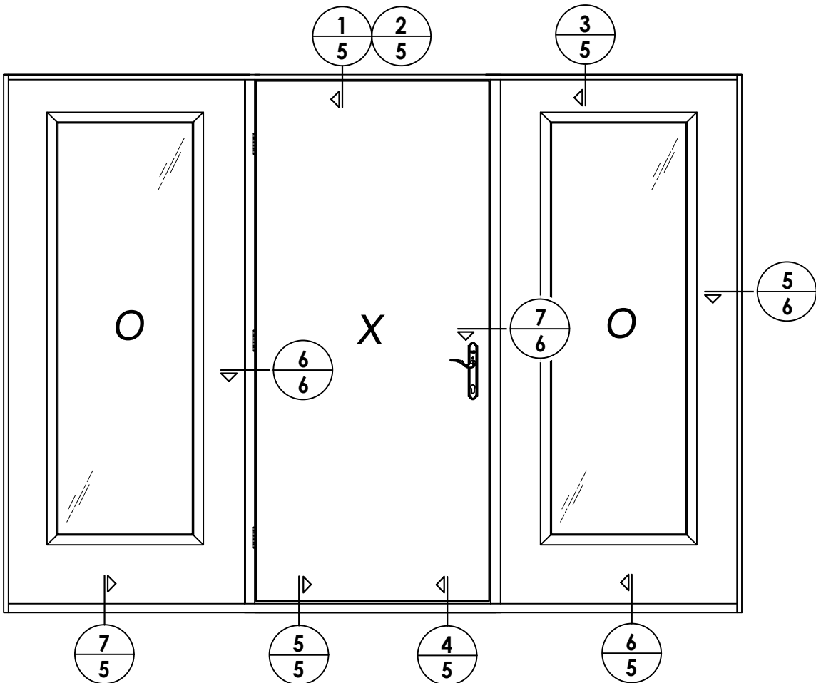
ELEVATION OXO
