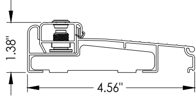
15 INSWING ADJUSTABLE THRESHOLD ZAILAA4565
