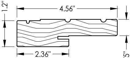
1 WOOD JAMB
